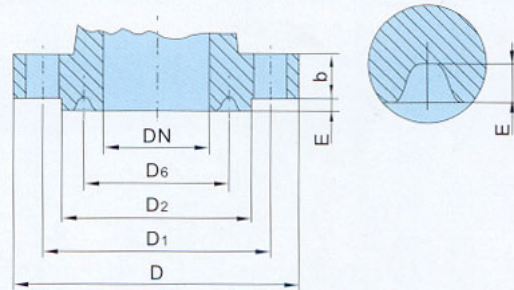
400Lb-600Lb(RJ)
